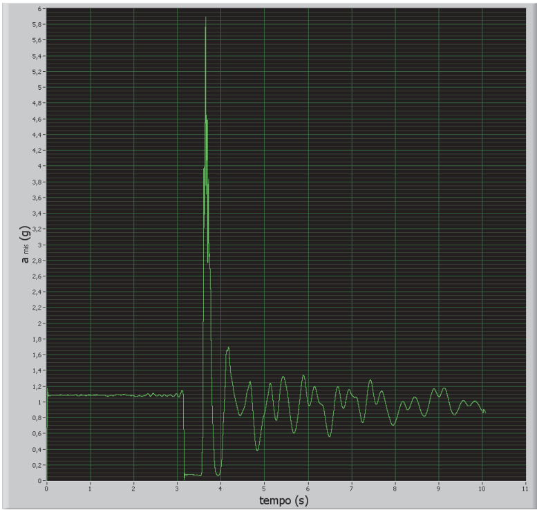
Figura A-41: Prova 80/1 F andamento di a_{\text{mis}} (g) rispetto al tempo [s]
