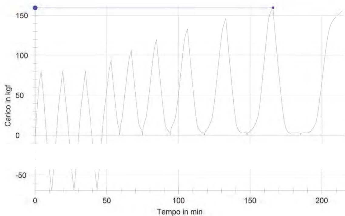
Figura 3-157 Curva carico-tempo
