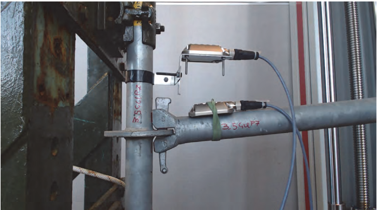
Figura 3-156 Foto fine prova
