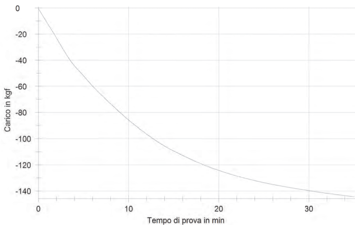
Figura 3-55 Curva carico-tempo.
