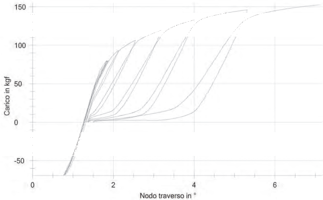
Figura 3-147 Curva carico – inclinazione traverso al nodo
