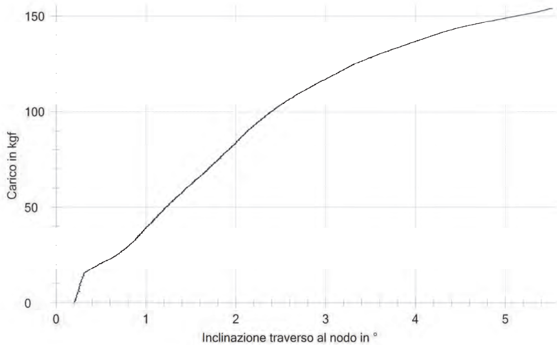
Figura 3-69 Curva carico – inclinazione traverso al nodo
