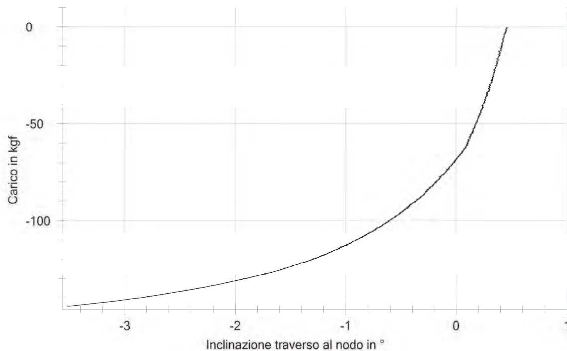
Figura 3-63 Curva carico – inclinazione traverso al nodo
