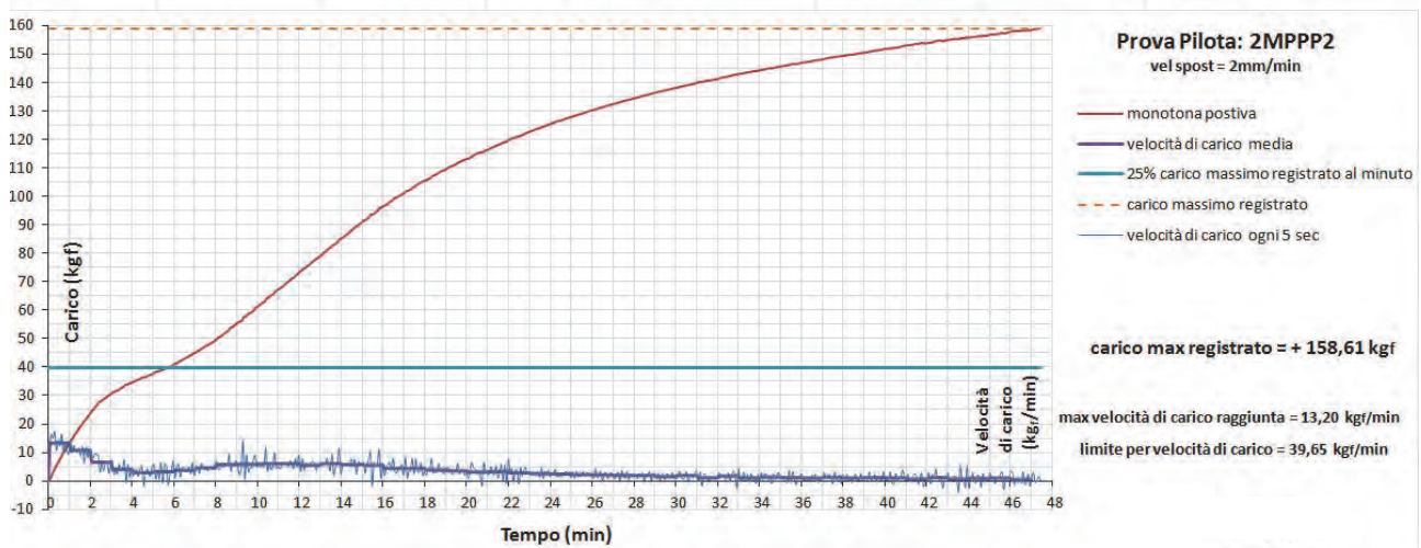
Figura 3-30 Curva carico-tempo. Velocità di carico media (kg/min). Limite per la velocità di carico calcolato in base al massimo carico registrato
